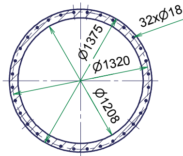
V-V ( 1 : 25 ) INLET FLANGE
